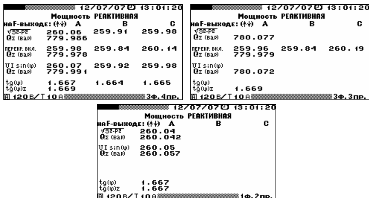
Рис. 4.7. Режим отображения реактивной мощности для различных схем включения
