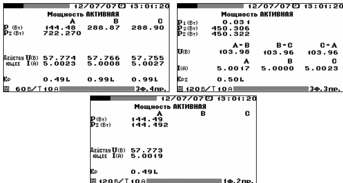
Рис. 4.6. Режим отображения активной мощности для различных схем включения
