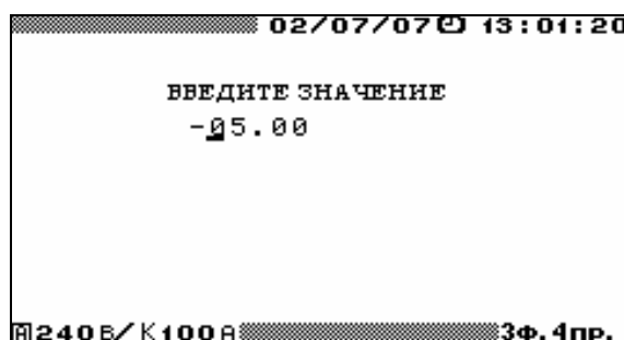
Рис. 4.74. Окно ввода новых значений уставок
