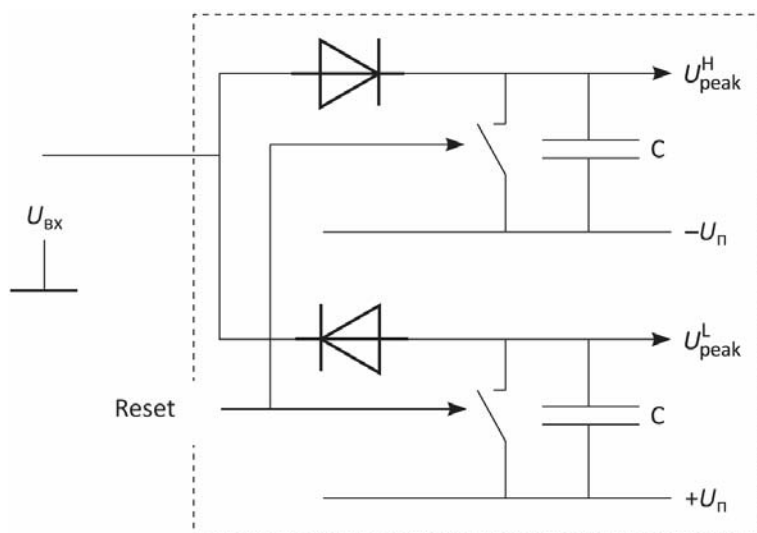
Рис. 4.50. Принцип обработки входного сигнала в режиме « ПИКОВЫЙ ДЕТЕКТОР »: U_{ВХ} — входное напряжение; f_s — частота дискретизации (12,8 кГц); Reset — сигнал сброса программного пикового детектора 1,25; 2,5; 5 или 10 с (выдается по программному таймеру в соответствии со значением « ВРЕМЯ УСРЕДНЕНИЯ », установленным в режиме « НАСТРОЙКИ » (см. п. 4.10.6)); U_{peak}^H — максимальное зафиксированное значение напряжения; U_{peak}^L — минимальное зафиксированное значение напряжения; C — элемент памяти программного пикового детектора; -U_{П} — минимально возможное напряжение; +U_{П} — максимально возможное напряжение
