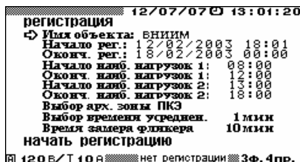
Рис. 4.16. Запрос на подтверждение начала регистрации ПКЭ
