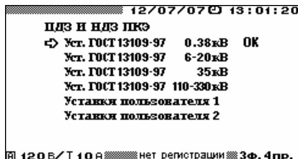
Рис. 4.15. Меню выбора типа уставок Прибора ЭМ-3.3Т1
