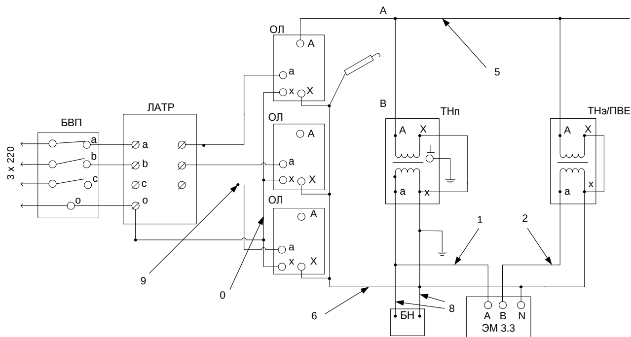
Рисунок Б.4 –Электрическая схема определения погрешностей однофазных заземляемых трансформаторов до 15/√3 кВ
