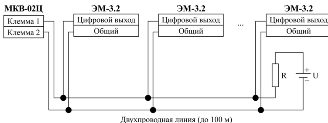
Рис. А.1. Схема подключения Модуля МКВ-02Ц к Приборам «Энергомонитор-3.2»
