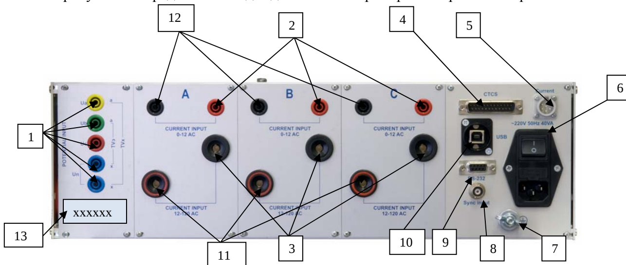
Рисунок 2.8 Вид задней панели прибора «Энергомонитор-3.1КМ»
