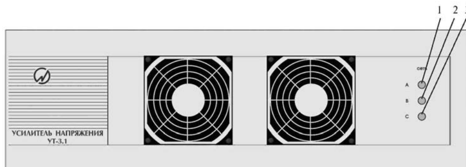
Рисунок 2.11 Вид лицевой панели усилителей напряжения «УН-3.1» 1,2,3 — индикаторы наличия питания на усилителе напряжения по фазам А, В, С.
