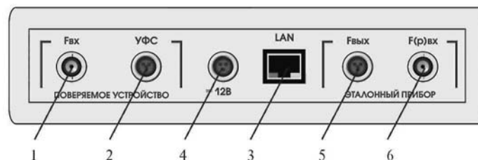
Рисунок 2.14 Передняя панель Преобразователя «ПТНЧ»
