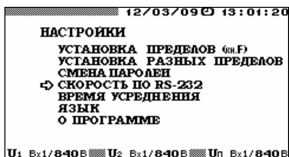
Рисунок 4.6.1 Меню настроек
