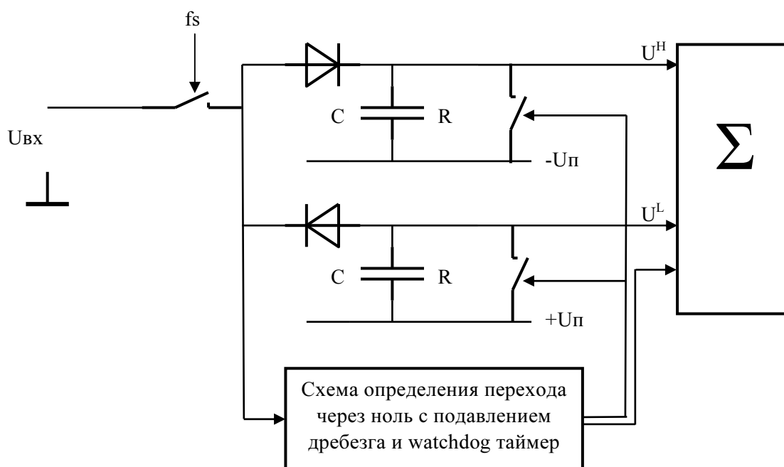
Рисунок 4.3.8 Принцип обработки входного сигнала в режиме 'Средняя амплитуда'
