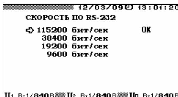
Рисунок 4.6.5 Меню выбора скорости обмена по интерфейсу RS-232
