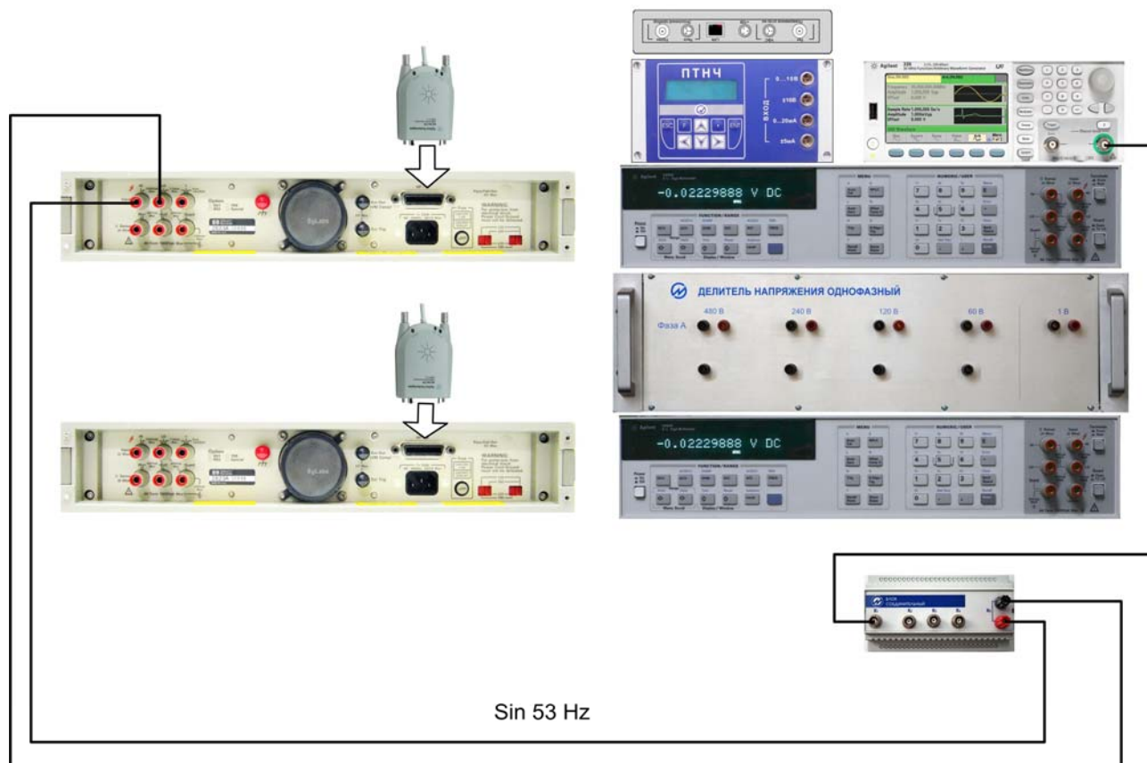
Рисунок А.7 - Схема цепи автокалибровки по частоте. НЧ – красный; ЛО – чёрный.
