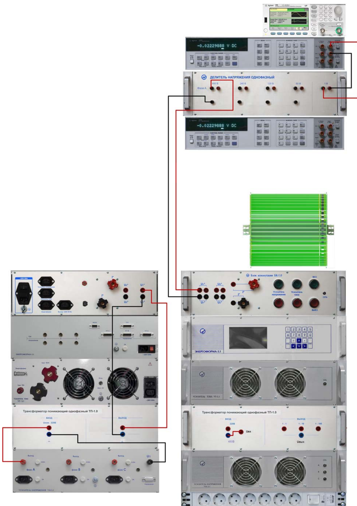
Рисунок А.4 - Схема измерительной цепи напряжения 480 В
