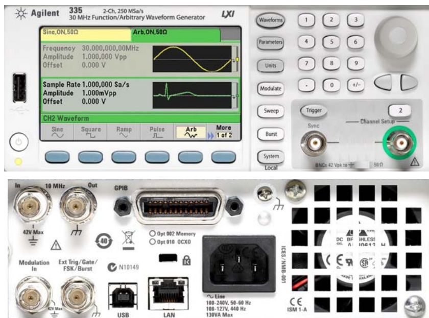
Рисунок 2.16. Генератор сигналов произвольной формы "33521В"
